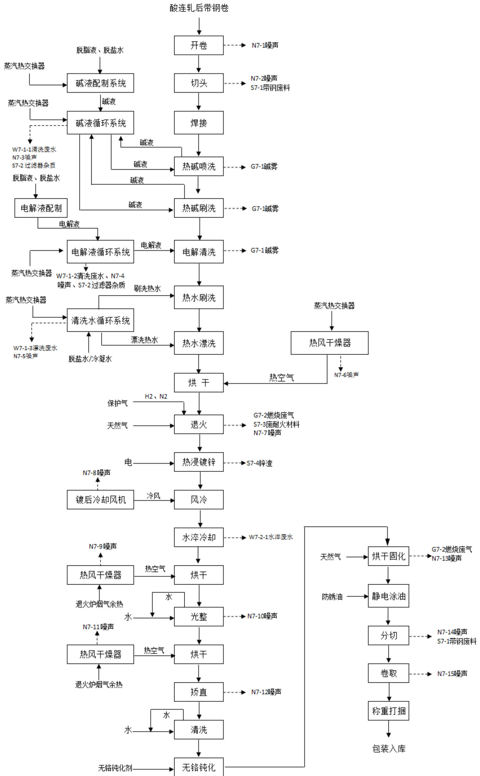
图3.5-9 连续热镀锌机组工艺流程及产污环节图
