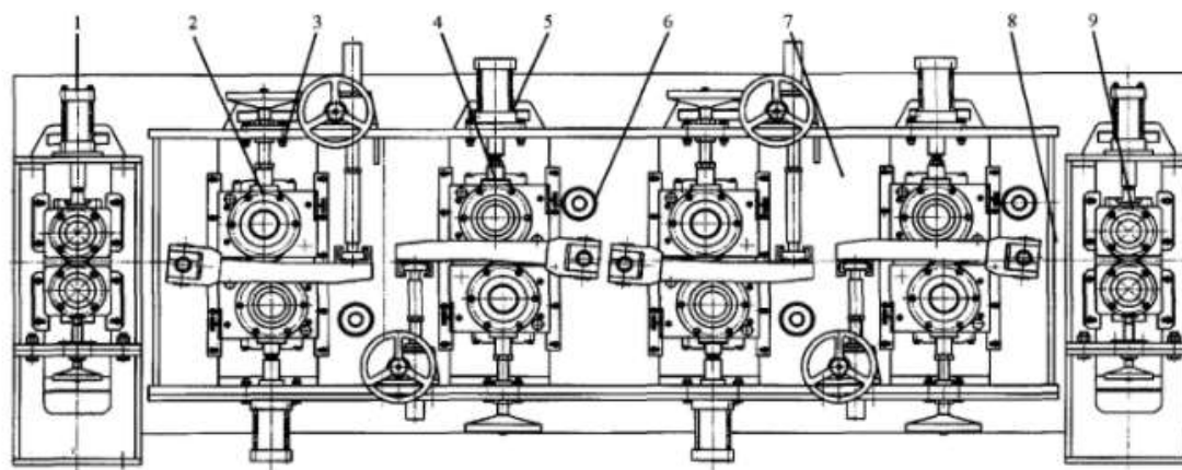
1—入口挤干辊;2—下刷辊;3—上支撑辊;4—上刷辊;5—下支撑辊;6—喷淋管;7—槽体;8—钢带;9—出口挤干辊
