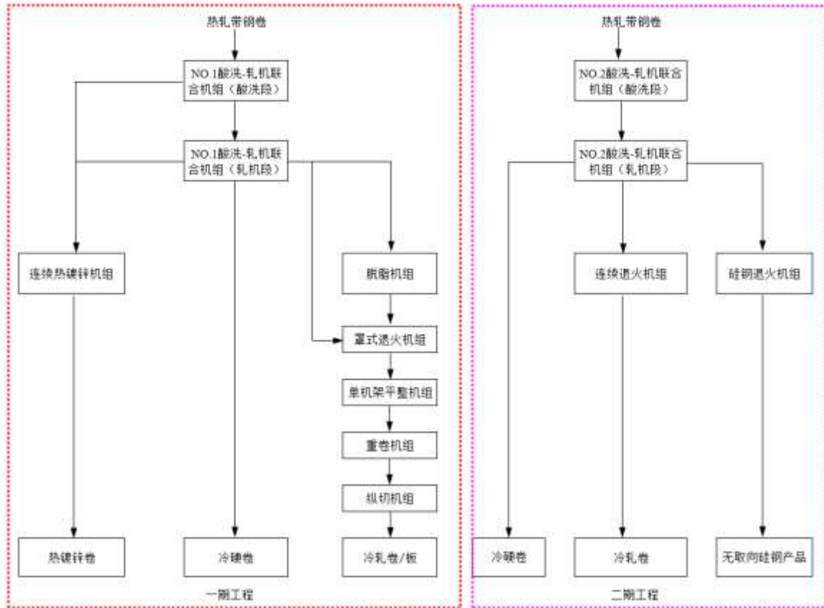
图3.5-1 本项目总体生产工艺方案图
