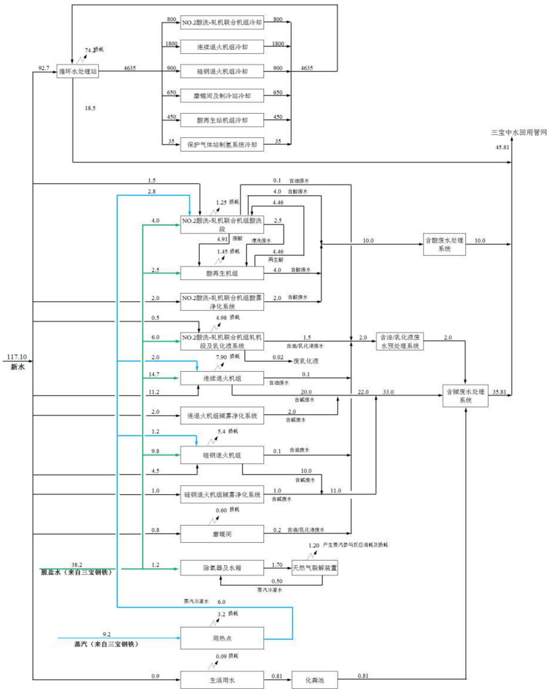
图 3.6-6 二期工程水平衡图 (单位: t/h)
