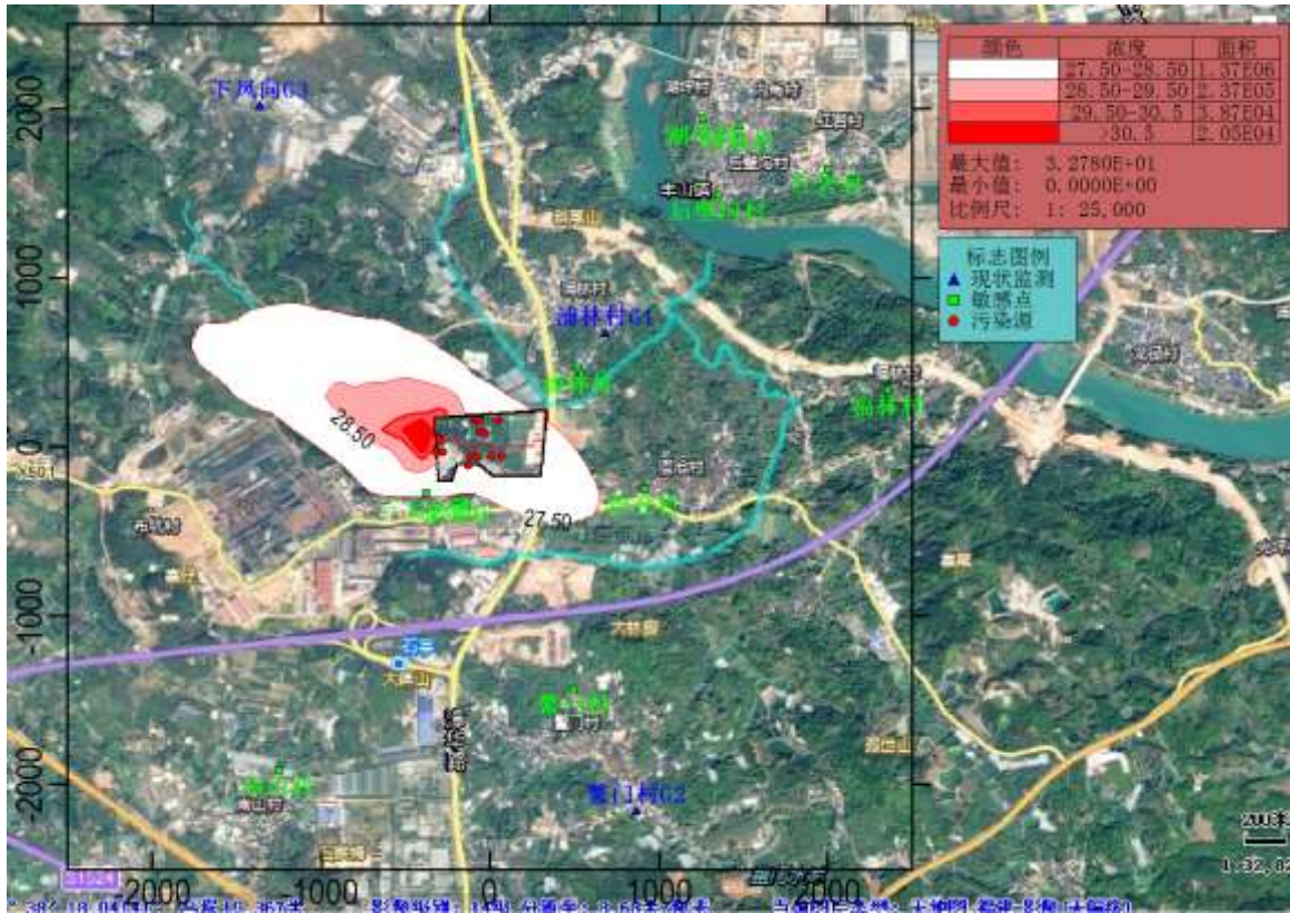
图 5.2.8-34 总体工程 NO x 年均浓度分布图 (µg/m 3 )
