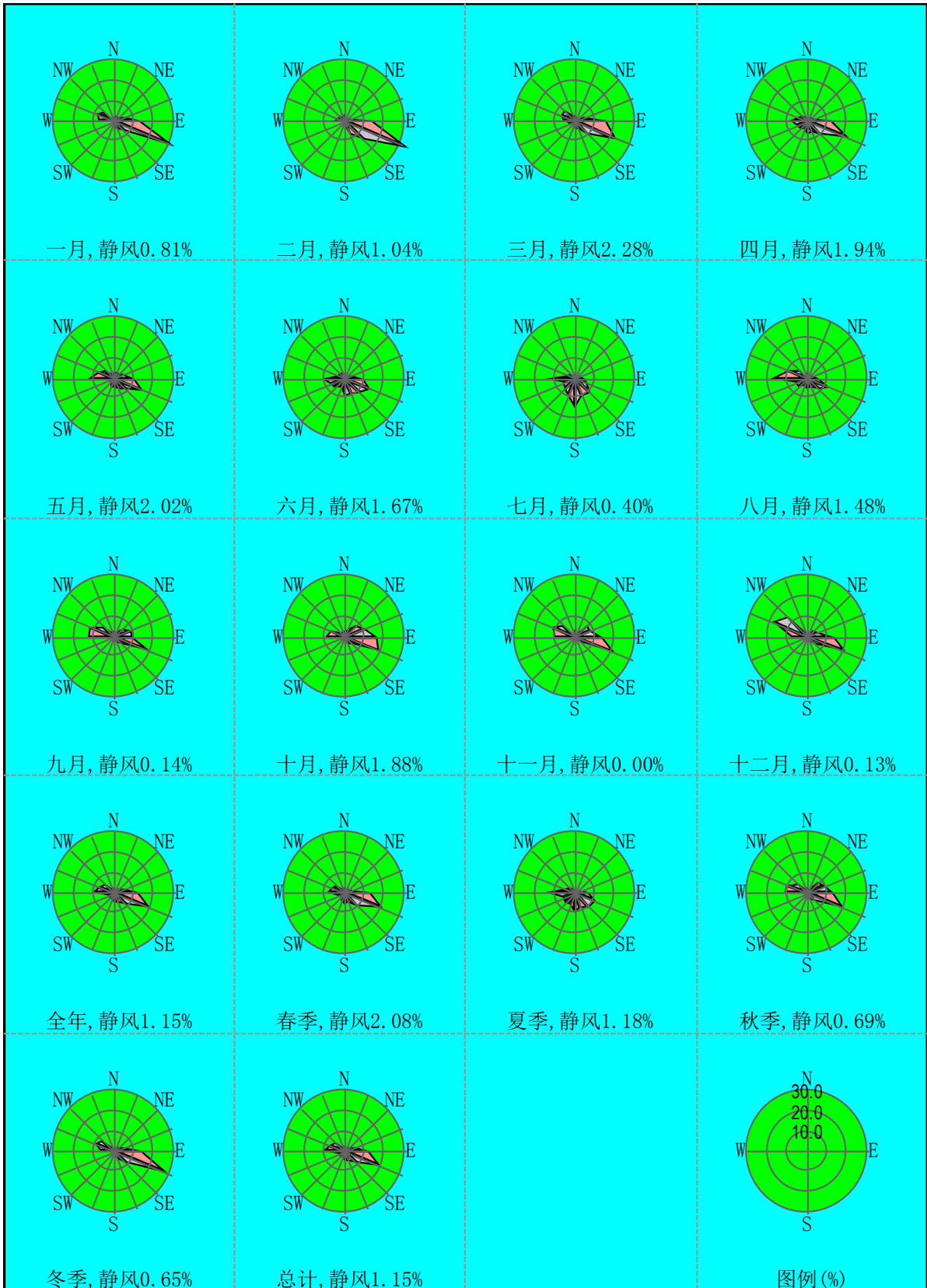
图 5.2.2-4 2019 年长泰县风频玫瑰图
