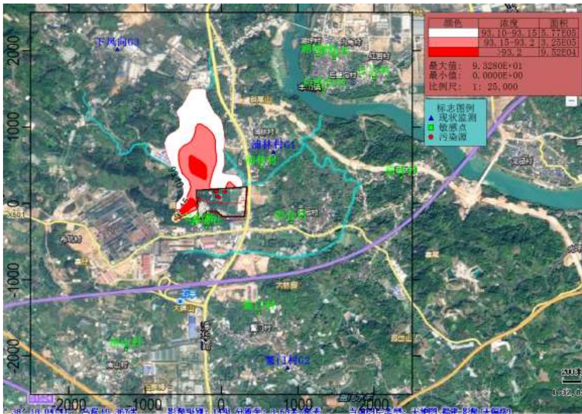
图 5.2.8-29 一期工程 PM 10 保证率日均浓度分布图 (μg/m 3 )
