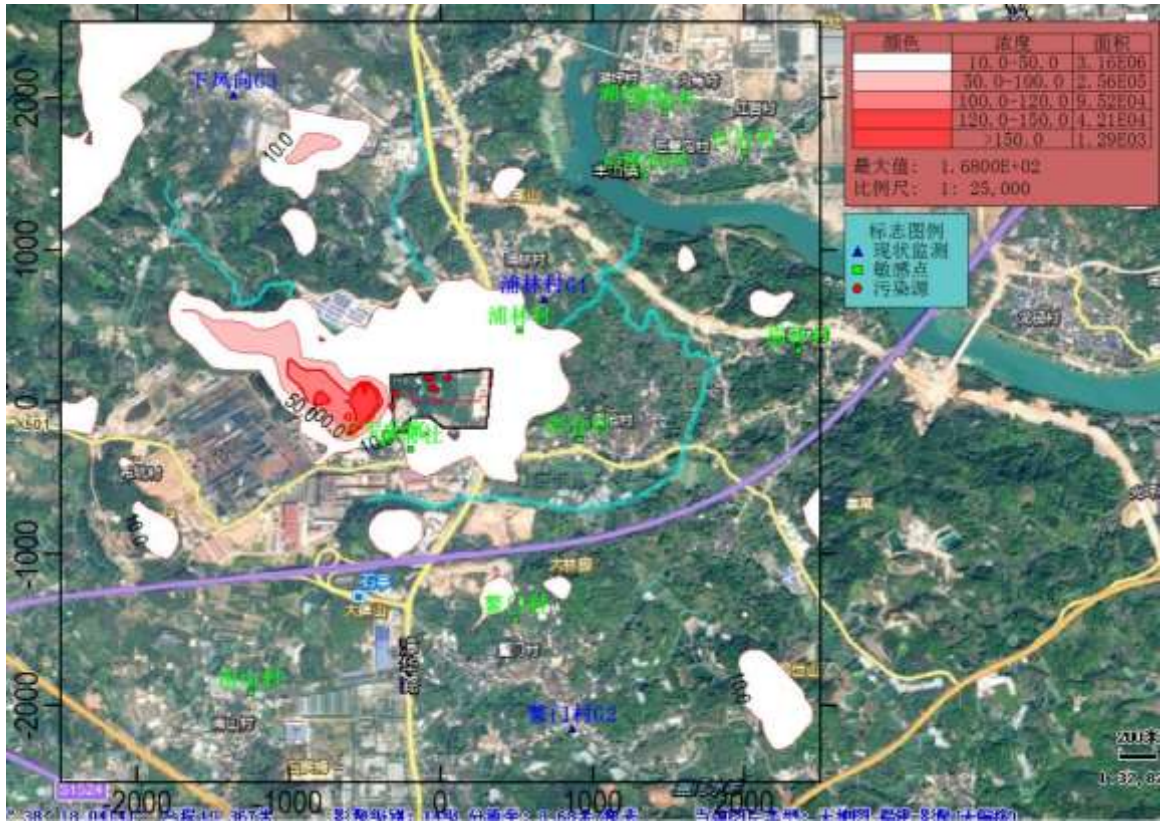
图 5.2.8-4 一期工程 NO x 小时浓度贡献分布图 ( \mu\text{g}/\text{m}^3 )
