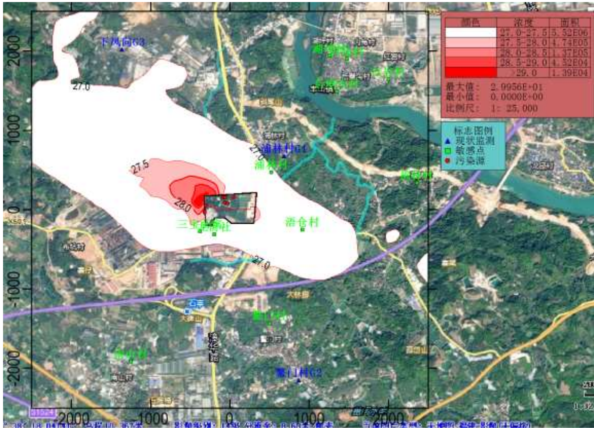
图 5.2.8-28 一期工程 NO x 年均浓度分布图 (μg/m 3 )
