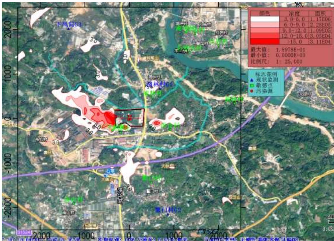
图 5.2.8-23 总体工程 HCl 小时均浓度贡献分布图 ( \mu\text{g}/\text{m}^3 )
