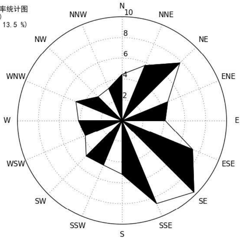
图 5.2.1-1 长泰气象站近 20 年风向玫瑰图
