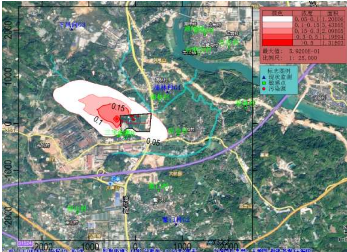
图 5.2.8-8 一期工程 PM 10 年均浓度贡献分布图 (µg/m 3 )
