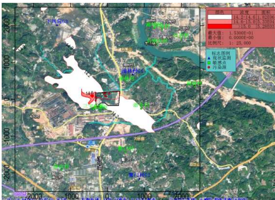
图 5.2.8-25 一期工程 SO 2 保证率日均浓度分布图
