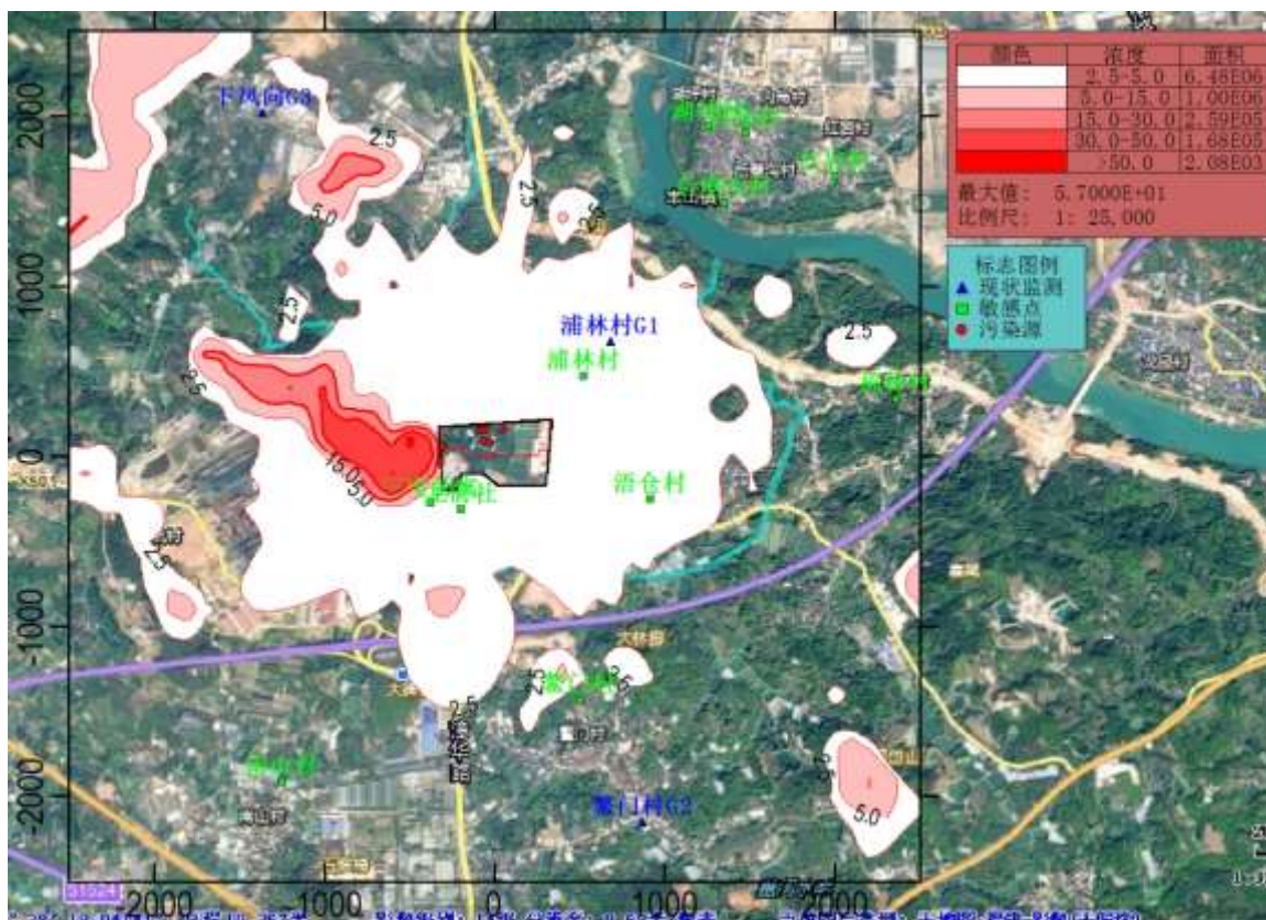
图 5.2.8-1 一期工程 SO 2 小时浓度贡献分布图 (μg/m 3 )
