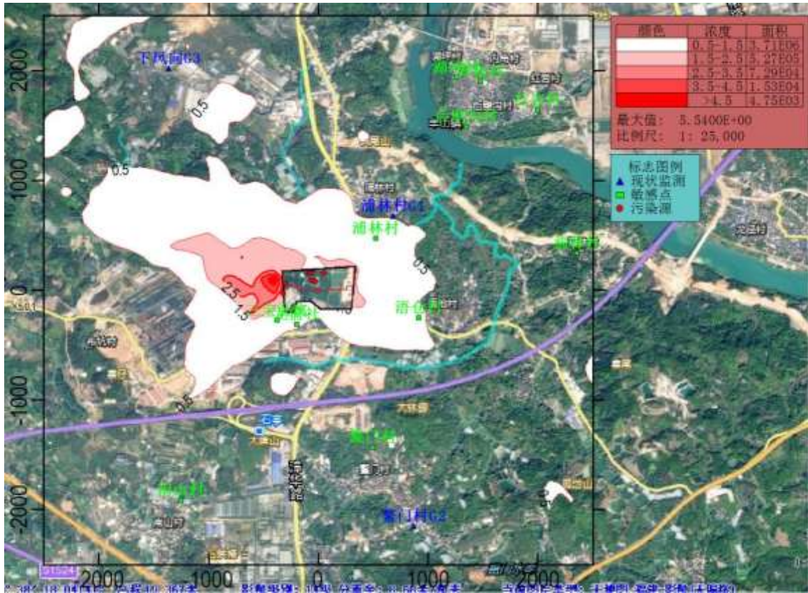
图 5.2.8-2 一期工程 SO 2 日均浓度贡献分布图 (µg/m 3 )
