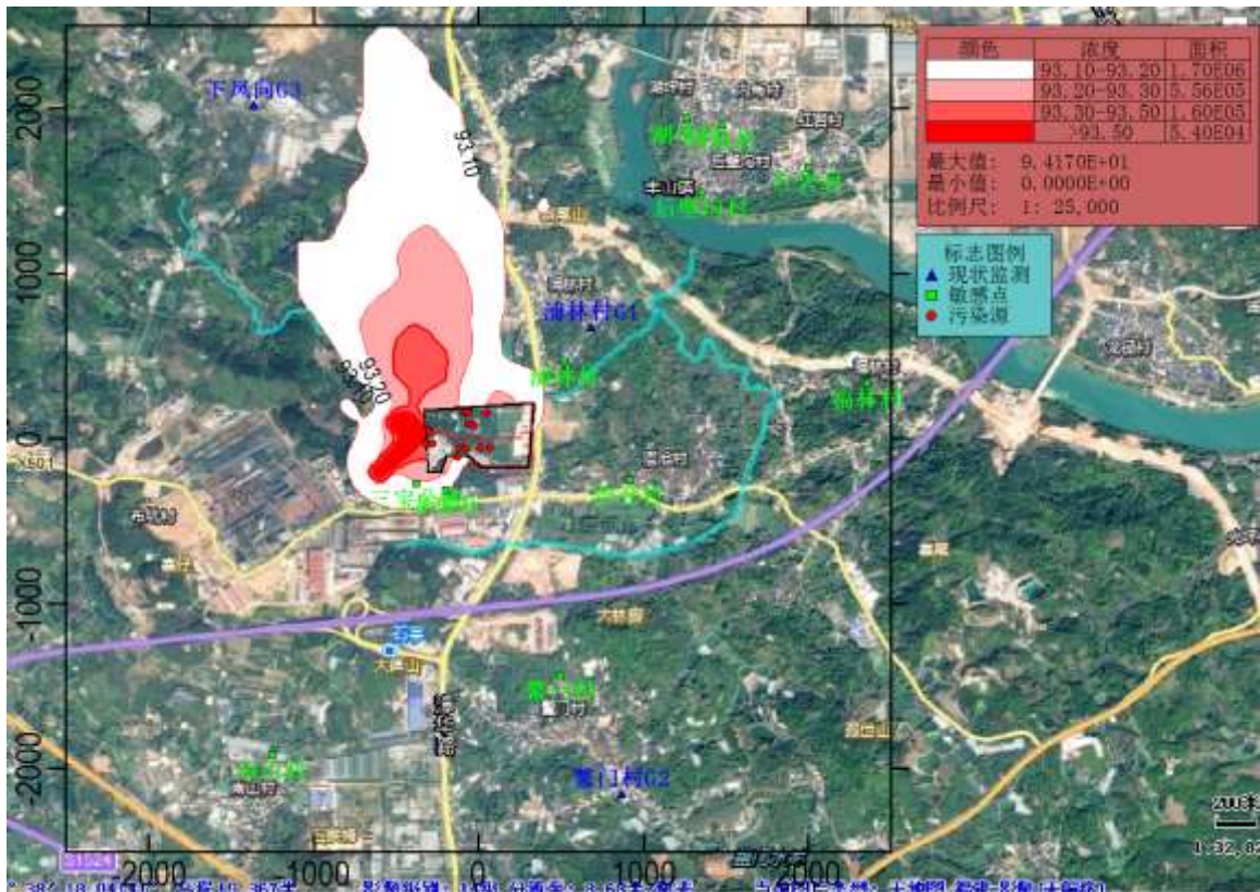
图 5.2.8-35 总体工程 PM 10 保证率日均浓度分布图 (µg/m 3 )
