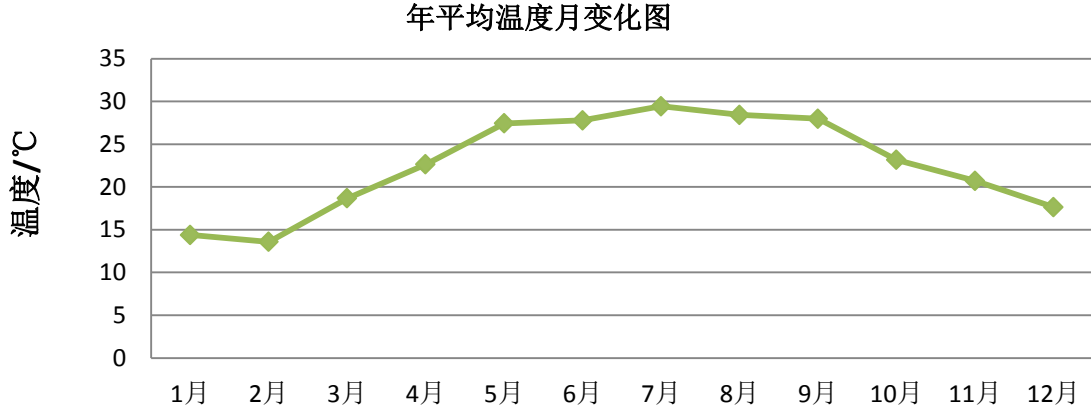
图 5.2.2-1 年平均温度月变化图
