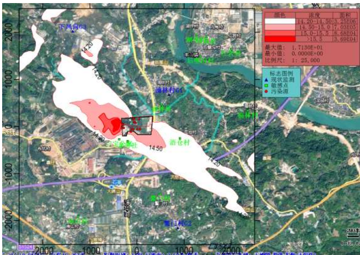
图 5.2.8-31 总体工程 SO 2 保证率日均浓度分布图 (µg/m 3 )
