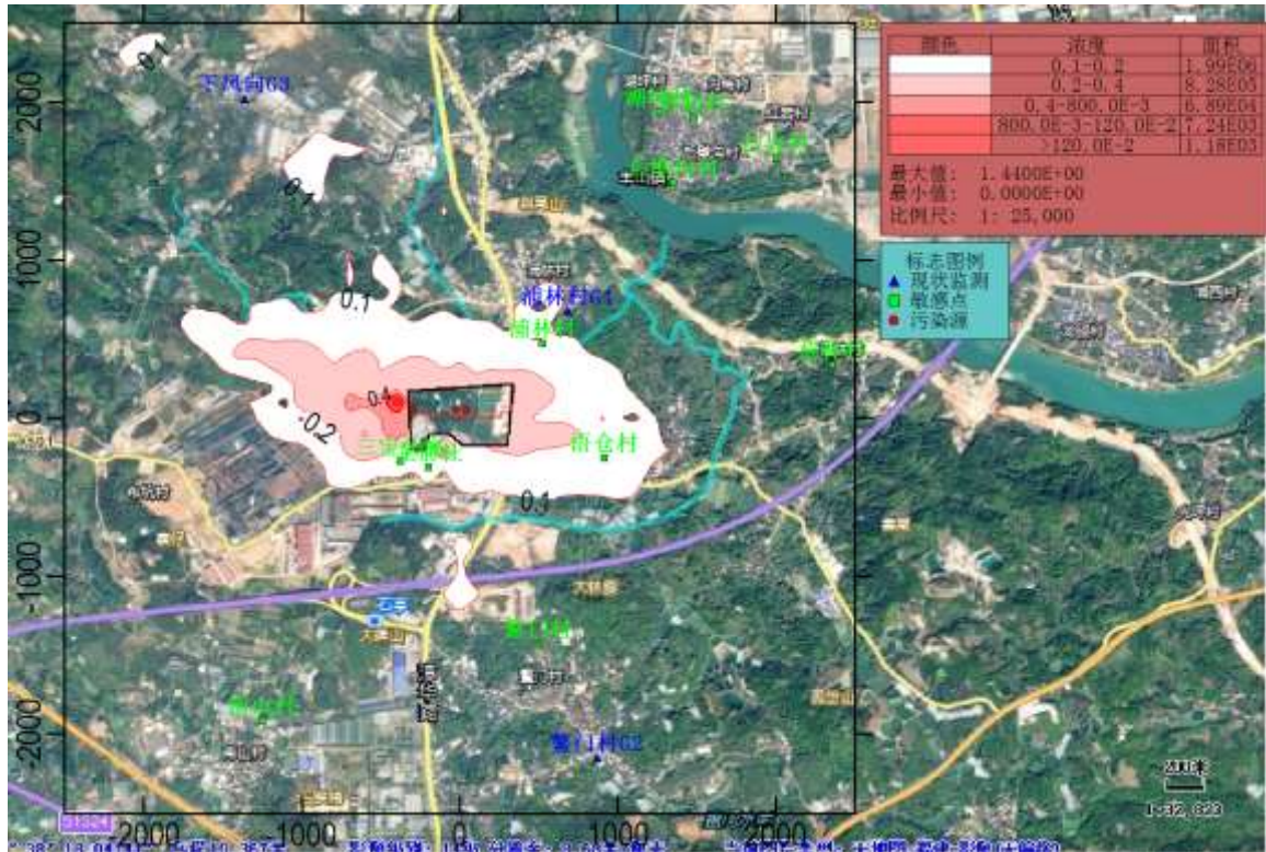
图5.2.8-12 一期工程HCl日均浓度贡献分布图 ( \mu\text{g}/\text{m}^3 )
