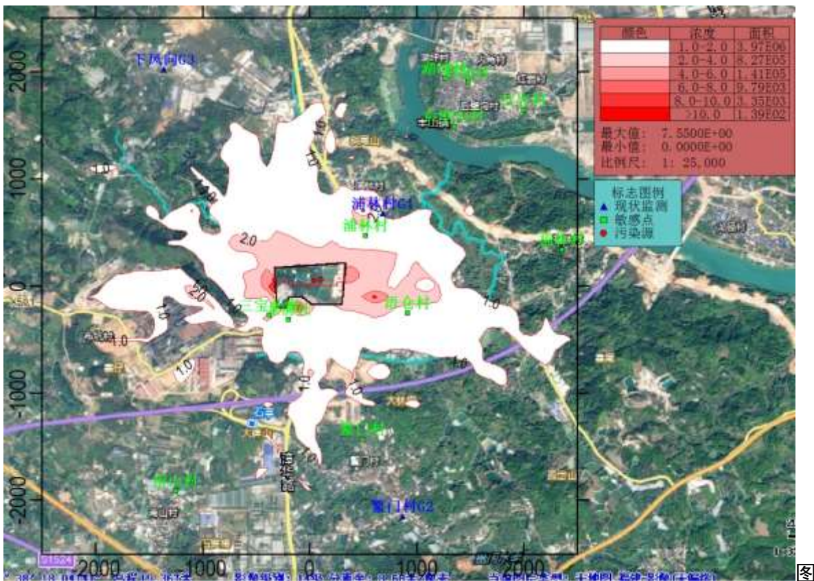
图 5.2.8-9 一期工程 TSP 日均浓度贡献分布图 (µg/m 3 )
