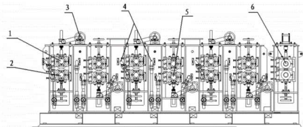
1-上刷洗辊 2-支撑辊 3-刷洗辊升降驱动电机 4-水喷管入口 5-下刷洗辊 6-挤干辊
