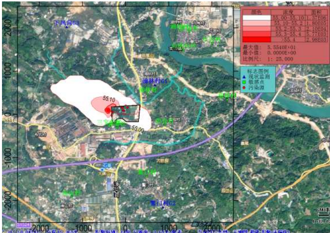
图 5.2.8-30 一期工程 PM 10 年均浓度分布图 (µg/m 3 )
