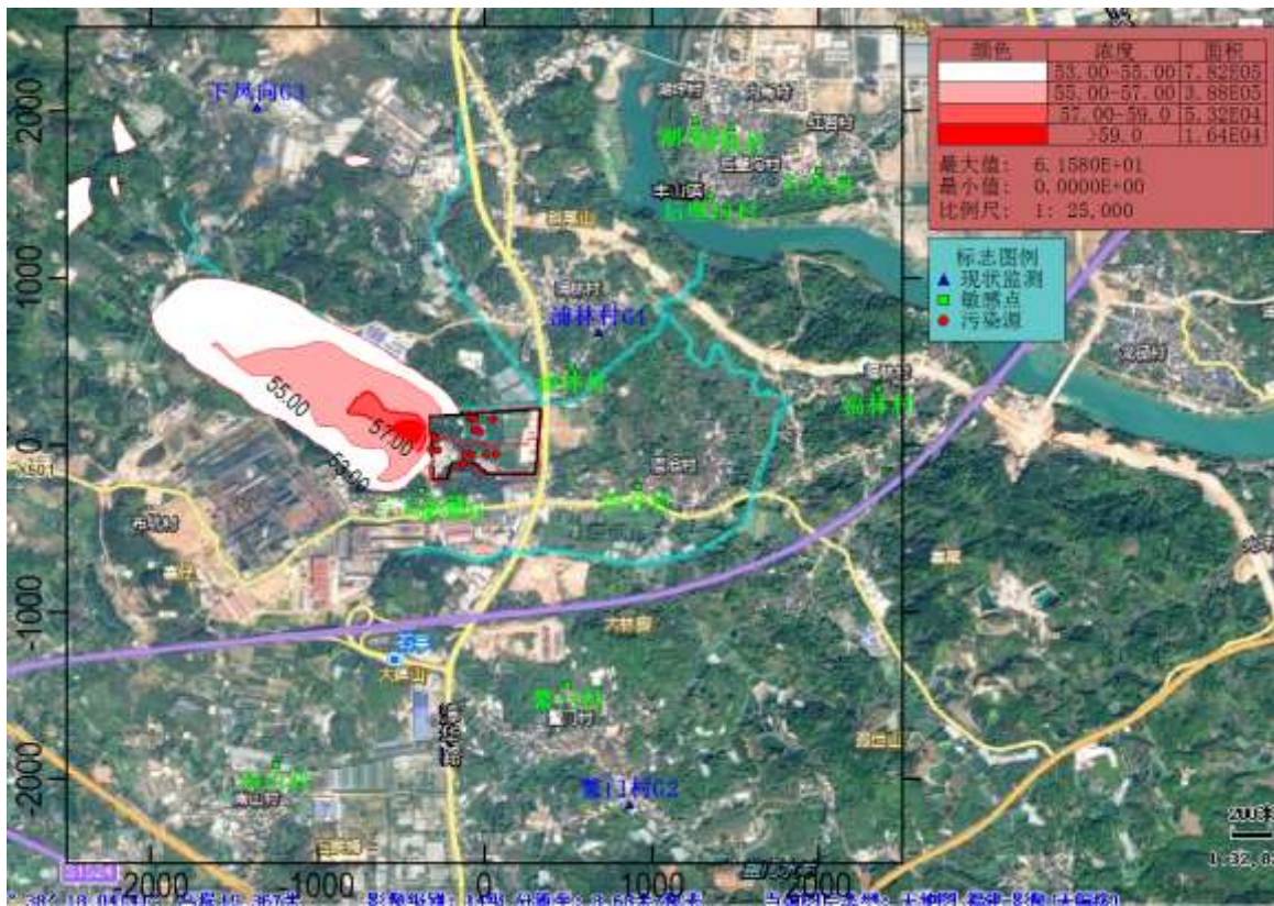
图 5.2.8-33 总体工程 NO x 保证率日均浓度分布图 (µg/m 3 )
