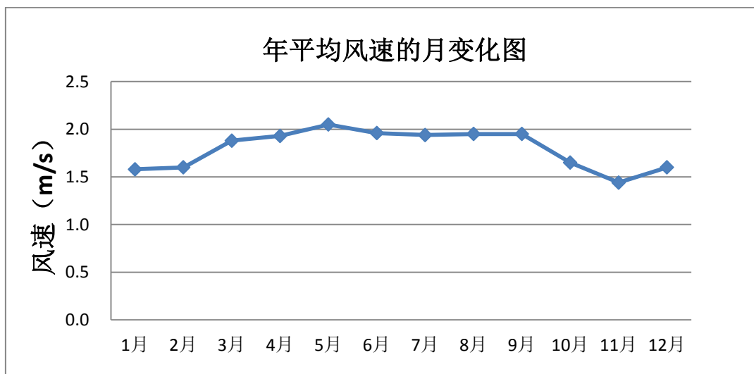
图 5.2.2-2 年平均风速的月变化图
