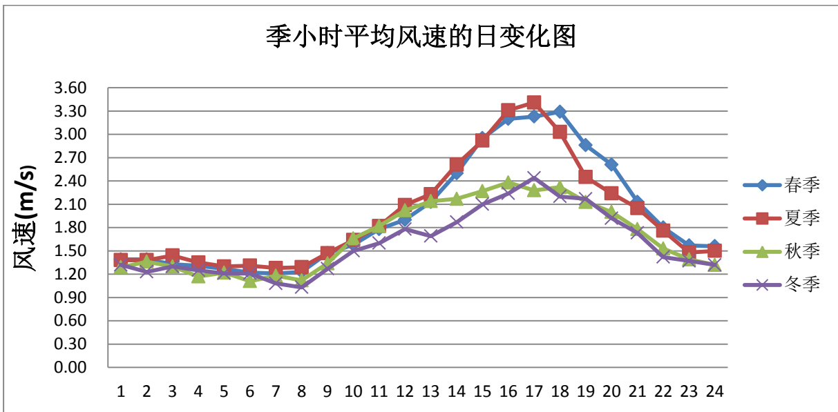
图 5.2.2-3 季小时平均风速日变化图
