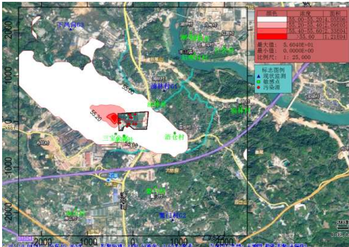
图 5.2.8-36 总体工程 PM 10 年均浓度分布图 (µg/m 3 )
