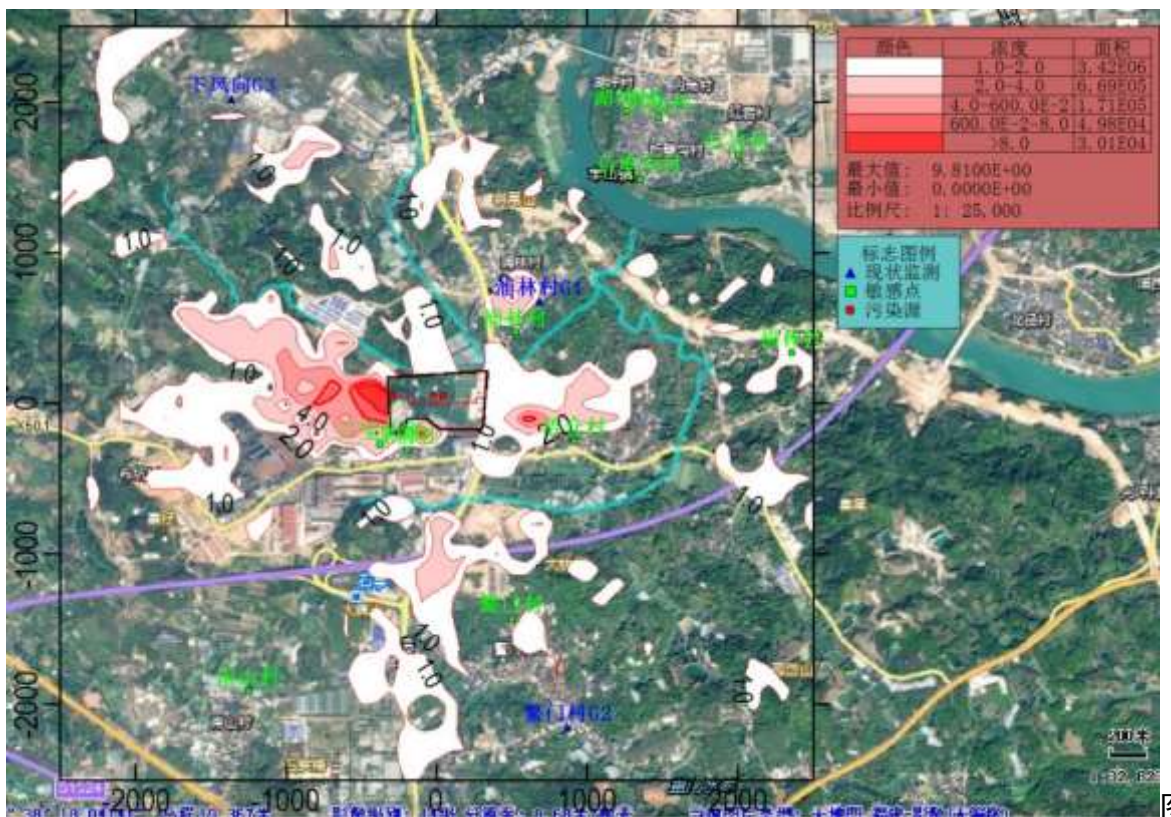
5.2.8-11 一期工程 HCl 小时浓度贡献分布图 ( \mu\text{g}/\text{m}^3 )
