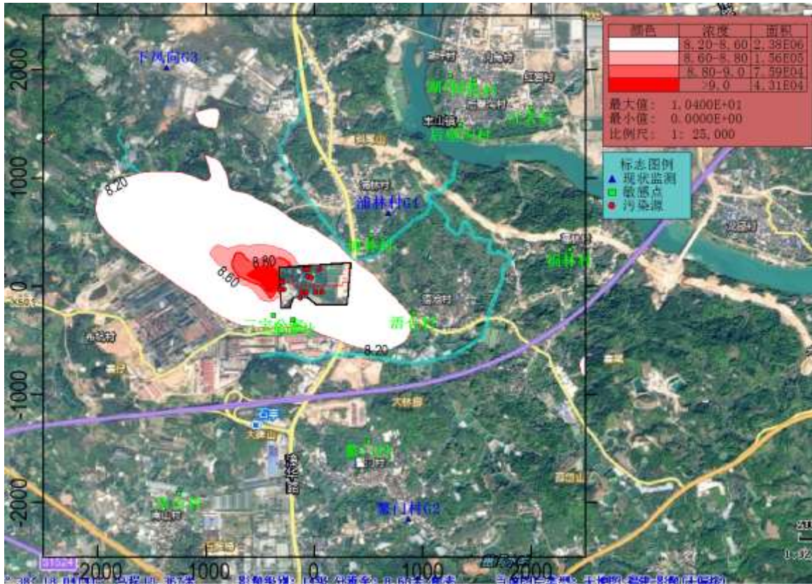
图 5.2.8-32 总体工程 SO 2 年均浓度分布图 (µg/m 3 )
