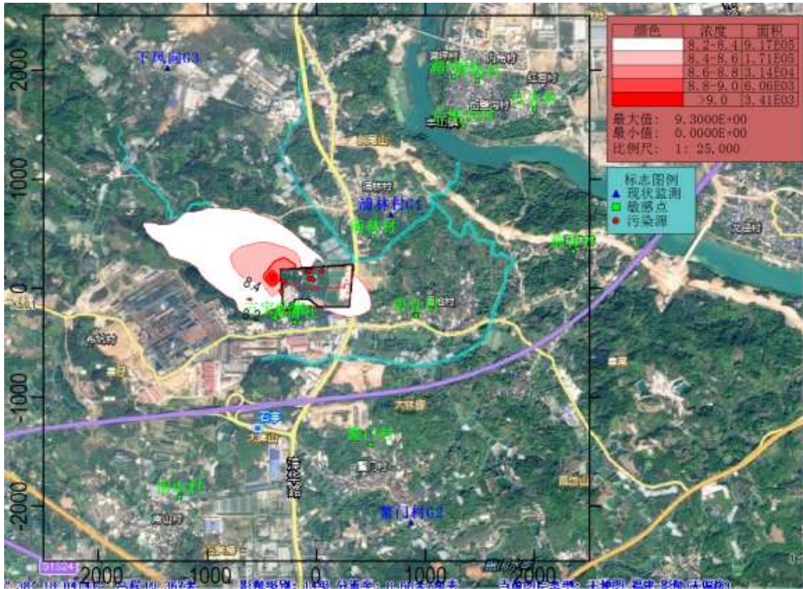
图 5.2.8-26 一期工程 SO 2 年均浓度分布图 (μg/m 3 )
