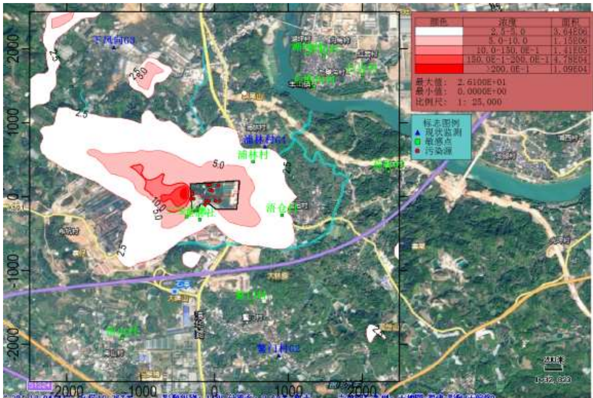
图 5.2.8-17 总体工程 NO x 日均浓度贡献分布图 (µg/m 3 )
