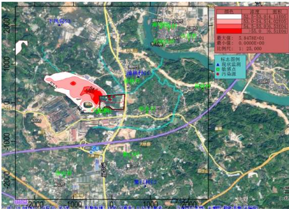
图 5.2.8-27 一期工程 NO x 保证率日均浓度分布图 (μg/m 3 )
