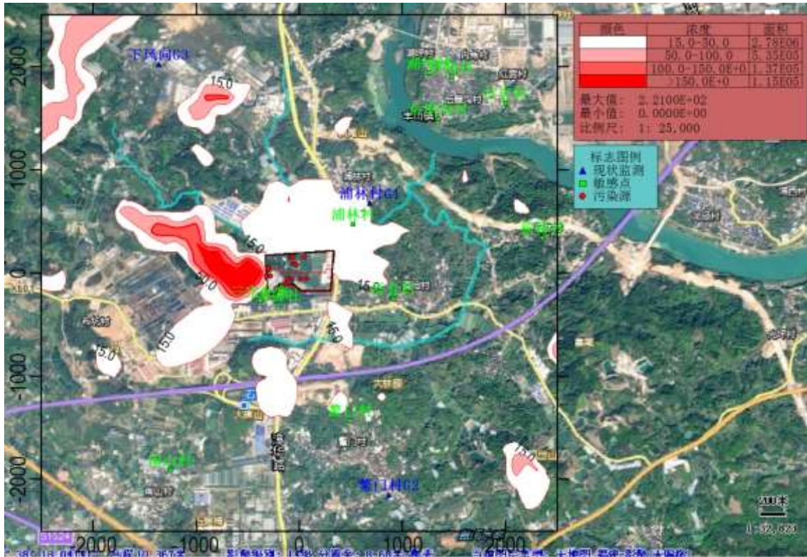
图 5.2.8-16 总体工程 NO x 小时浓度贡献分布图 (µg/m 3 )
