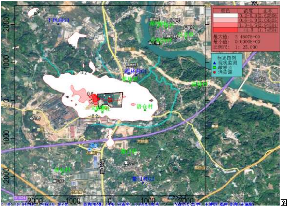
图 5.2.8-24 总体工程 HCl 日均浓度贡献分布图 ( \mu\text{g}/\text{m}^3 )
