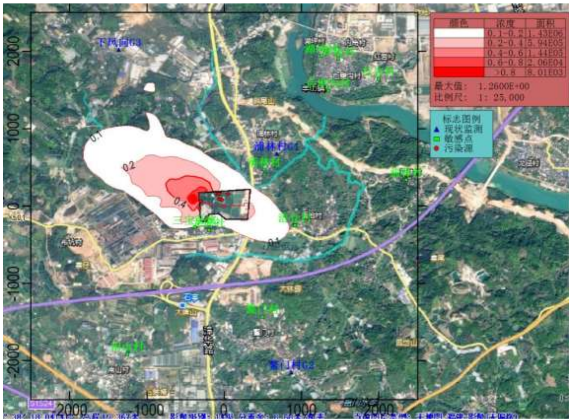
图 5.2.8-3 一期工程 SO 2 年均浓度贡献分布图 (µg/m 3 )
