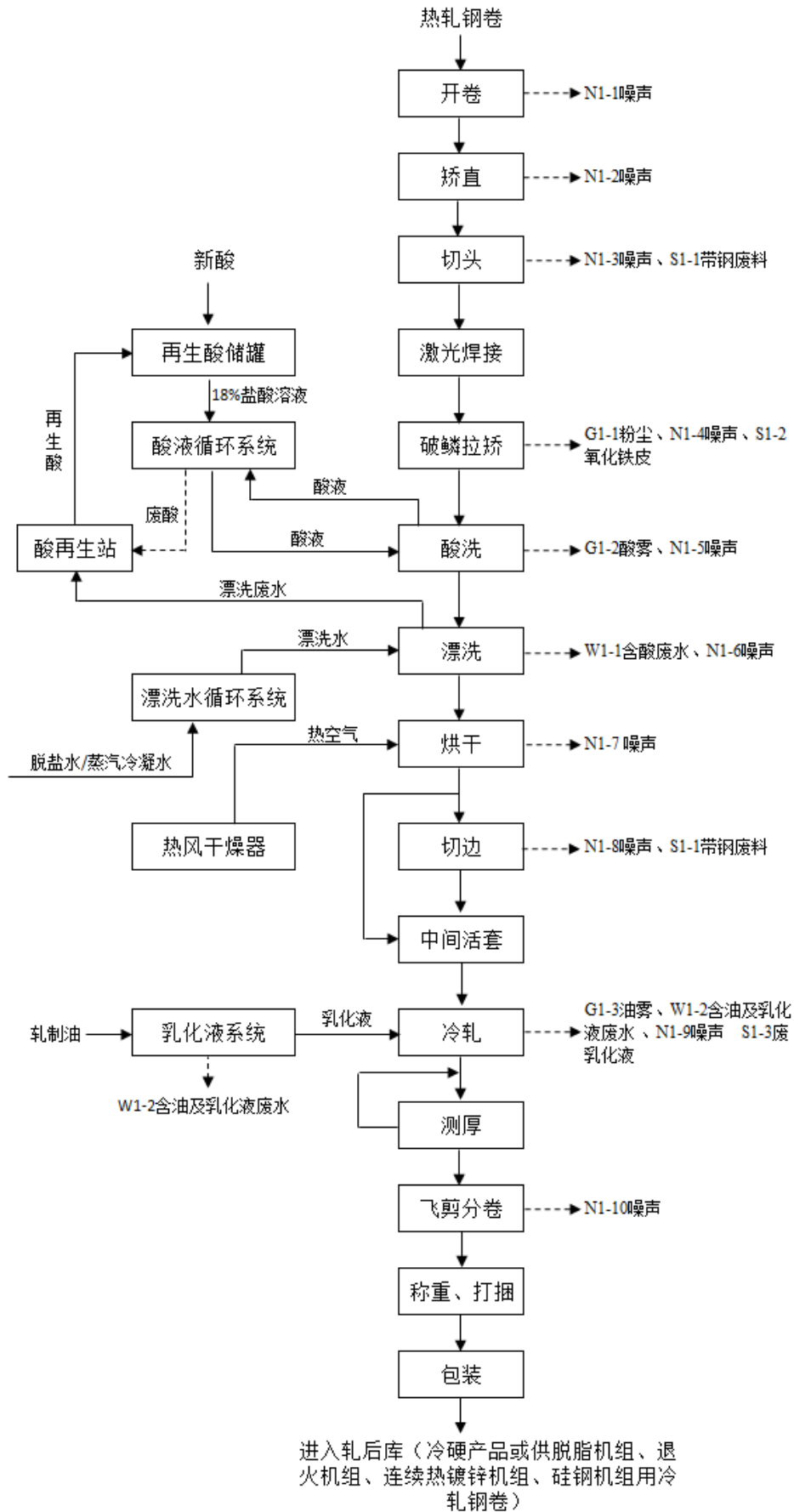
图 3.5-2 酸洗-轧机联合机组工艺流程及产污环节图
